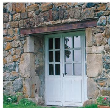
Borée, ouverture agrandie avec un linteau métallique droit qui permet la pose aisée d'une menuiserie vitrée. L'ancien cintre sert d'arc de décharge.
